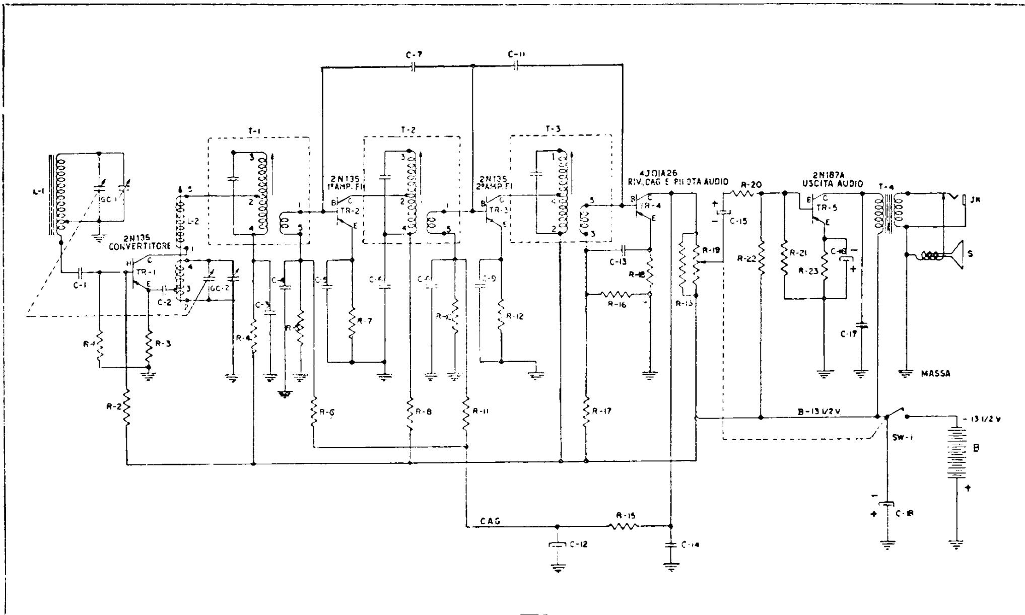
Fig. 8-4. - Radioricevitore portatile per onde medie a cinque transistori (Trav-ler mod. TR-250A). Si noti l'uso di un transistore al posto del diodo rivelatore.
